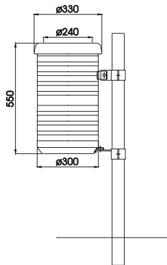
PALO DIAM. 60 DA INGHISARE
