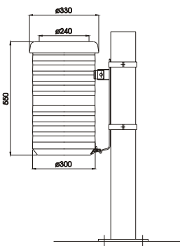
PALO DIAM. 120 CON PIASTRA
