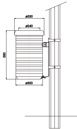
COLLARI SU PALI ESISTENTI A SEZIONE OTTAGONALE DIM.188-206-238
