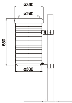
PALO DIAM. 60 CON PIASTRA
