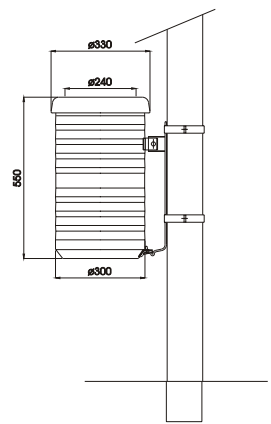
COLLARI SU PALI ESISTENTI DIAM.60-90-120-160-190-200-250
