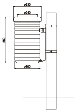
PALO DIAM. 120 DA INGHISARE
